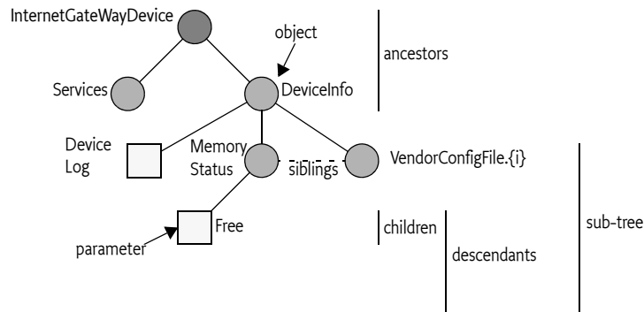
TR-069 Object and Parameter naming relative to the parameter MemoryStatus
